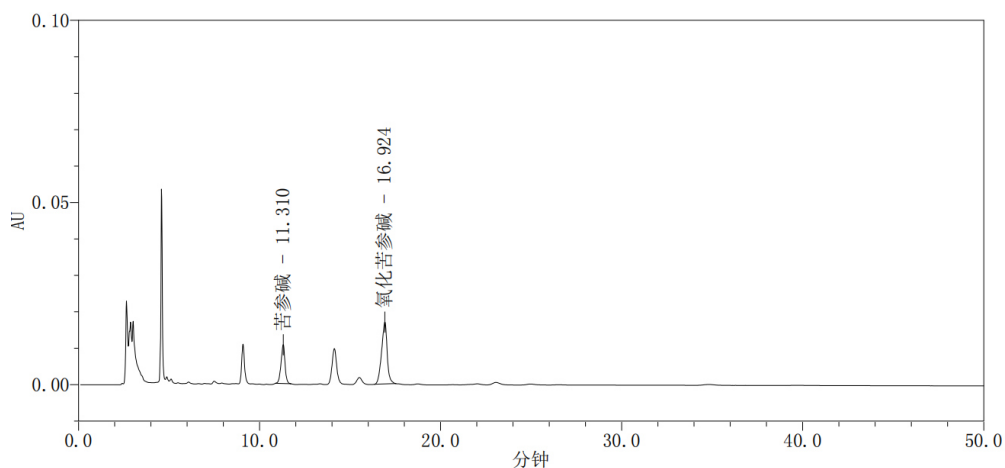
供试品溶液色谱图：
