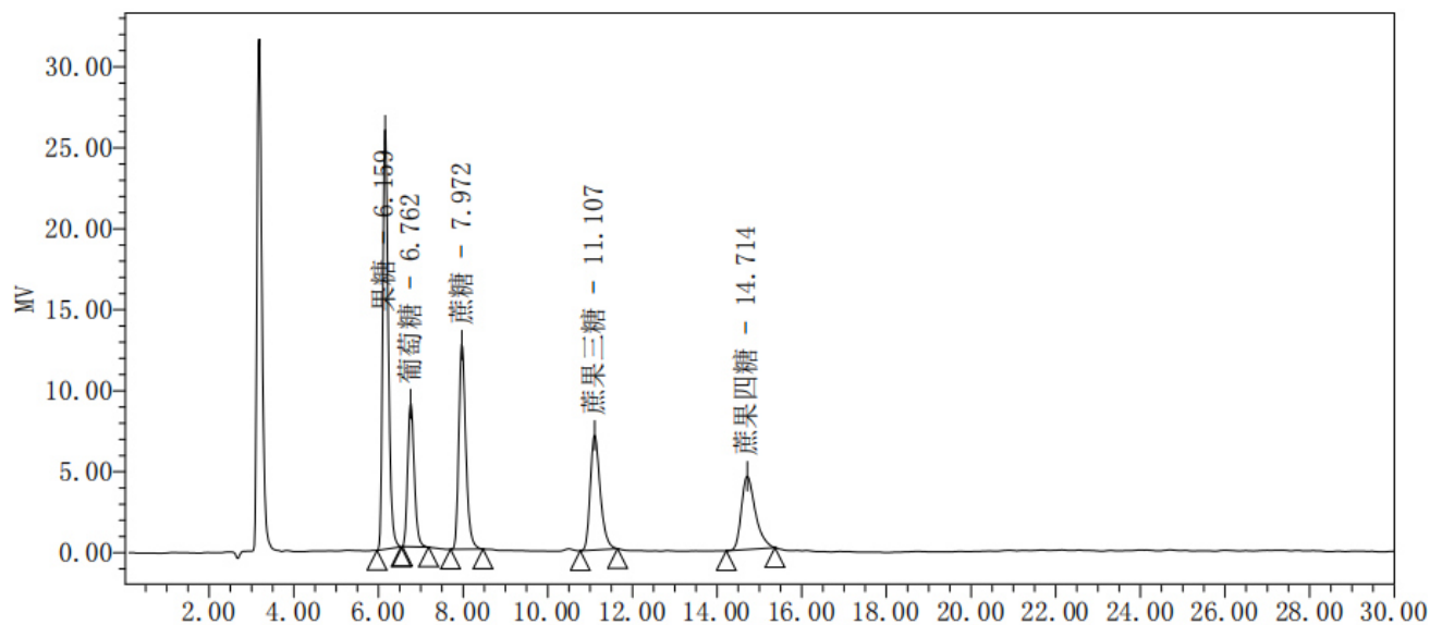
对照品溶液色谱图：
