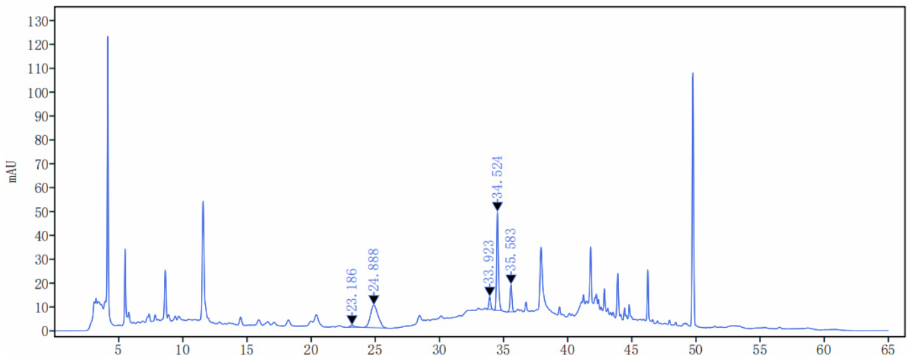
供试品溶液色谱图 (UV 240nm: 莫诺苷、马钱苷):
