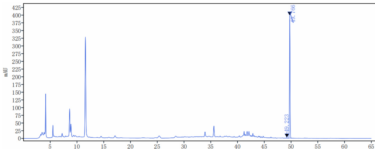
供试品溶液色谱图 (UV 274 nm: 丹皮酚):
