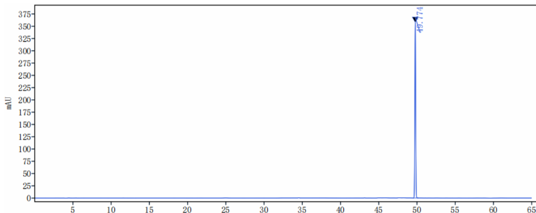
对照品溶液色谱图 (UV 274 nm: 丹皮酚):
