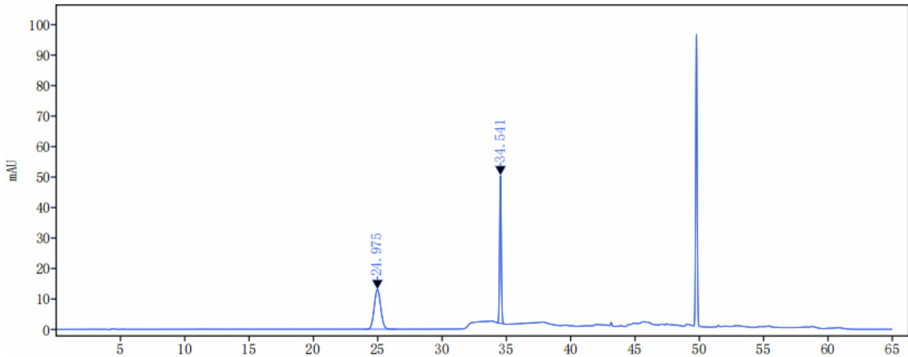
对照品溶液色谱图 (UV 240nm: 莫诺苷、马钱苷):
