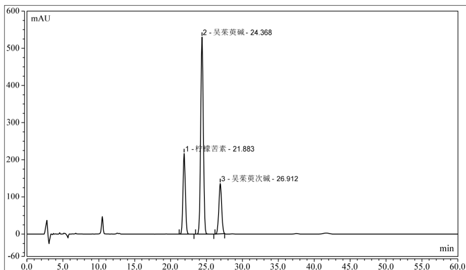
对照品溶液色谱图：
